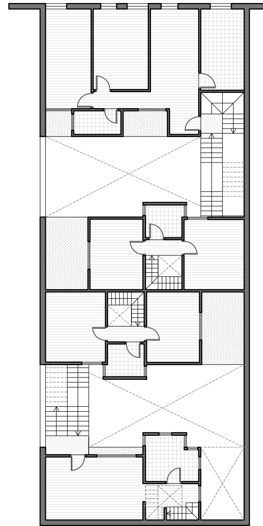
PLANTA 2º PAVIMENTO
