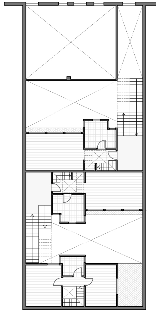
PLANTA 1º PAVIMENTO
