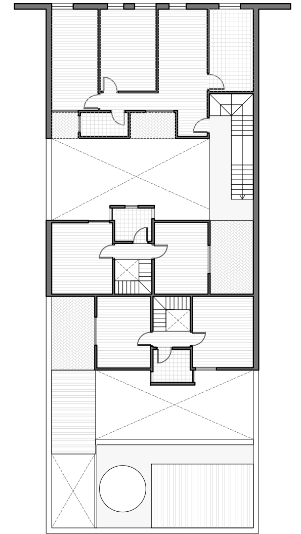
PLANTA 4º PAVIMENTO
